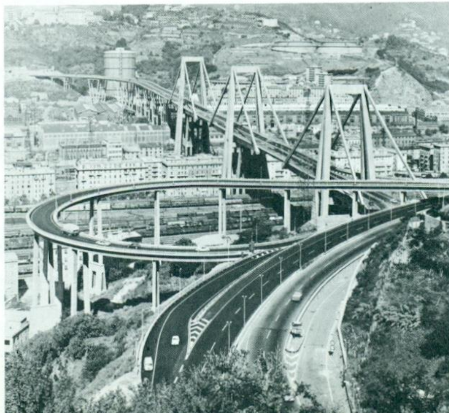
58. Riccardo Morandi: Viaduct above Polcevera, Genoa.
